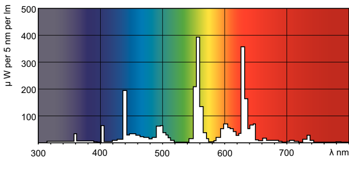
Barwa Światła /840
