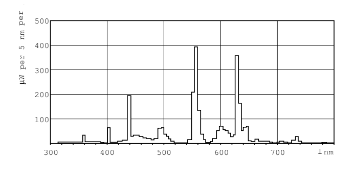
Barwa Światła /840
